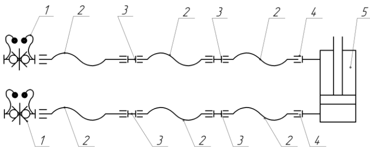
Рисунок 4 Схема гидравлики
